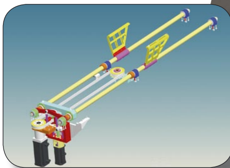
Azionamento spingitori. Pusher arm operating system. Groupe mécanique actionneur des bras de transfert. Greifarmantrieb. Accionamiento empujador.
