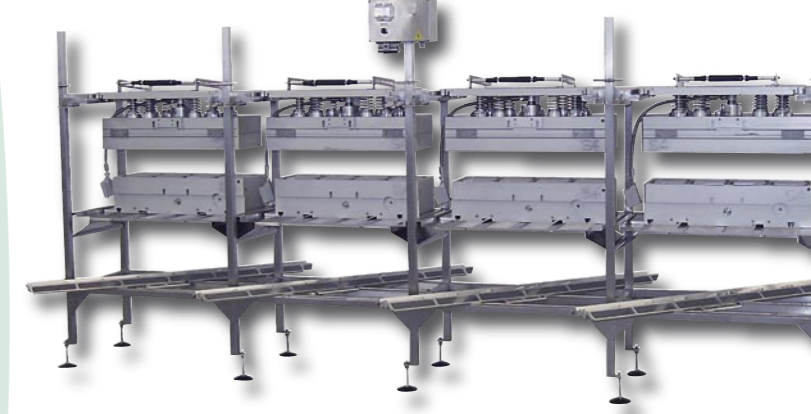
Carrello sostituzione stampi. Sealing tool change over trolley with top tool turn over device. Chariot pour substitution des outils d'operculage. Werkzeugwechselwagen mit Drehvorrichtung. Carrito sustitución moldes.
