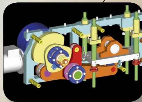
Azionamento stampo chiusura. Mechanical cam operating system - sealing tool closing. Démontage rapide des tapis d'entrée avec vérins tendeurs. Antrieb Verschlusswerkzeug. Accionamiento molde de cerrado.
